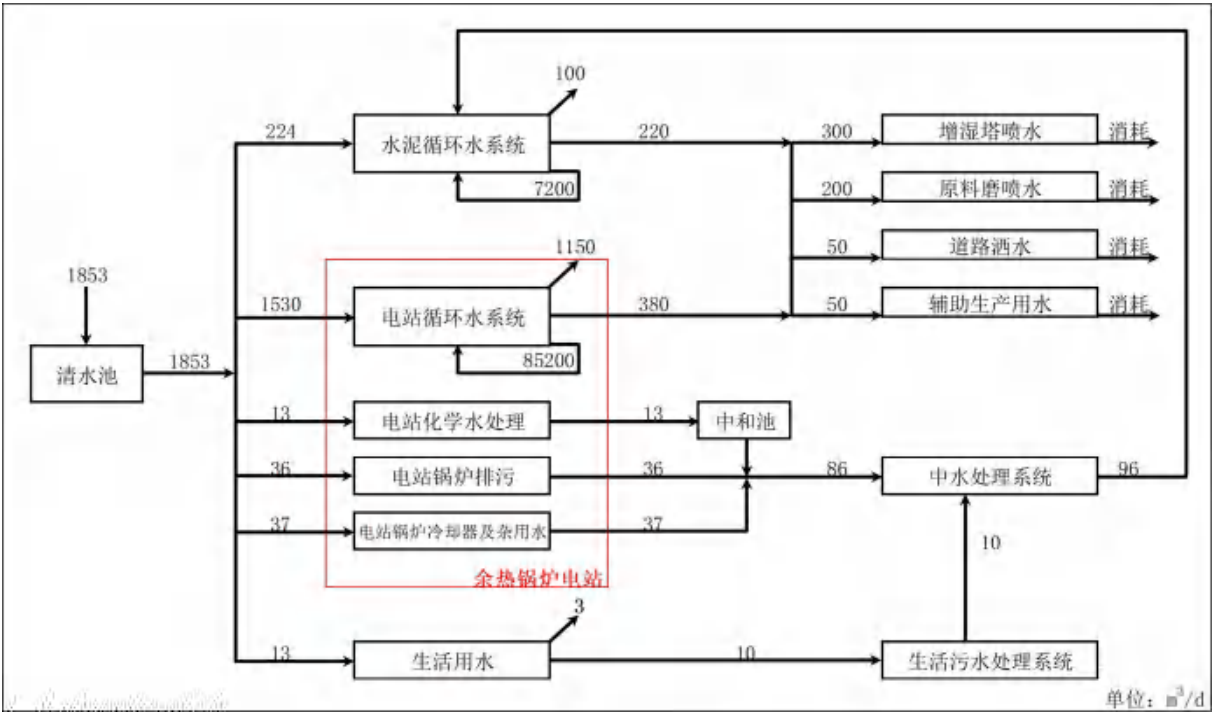
图 3—4 水量平衡图
