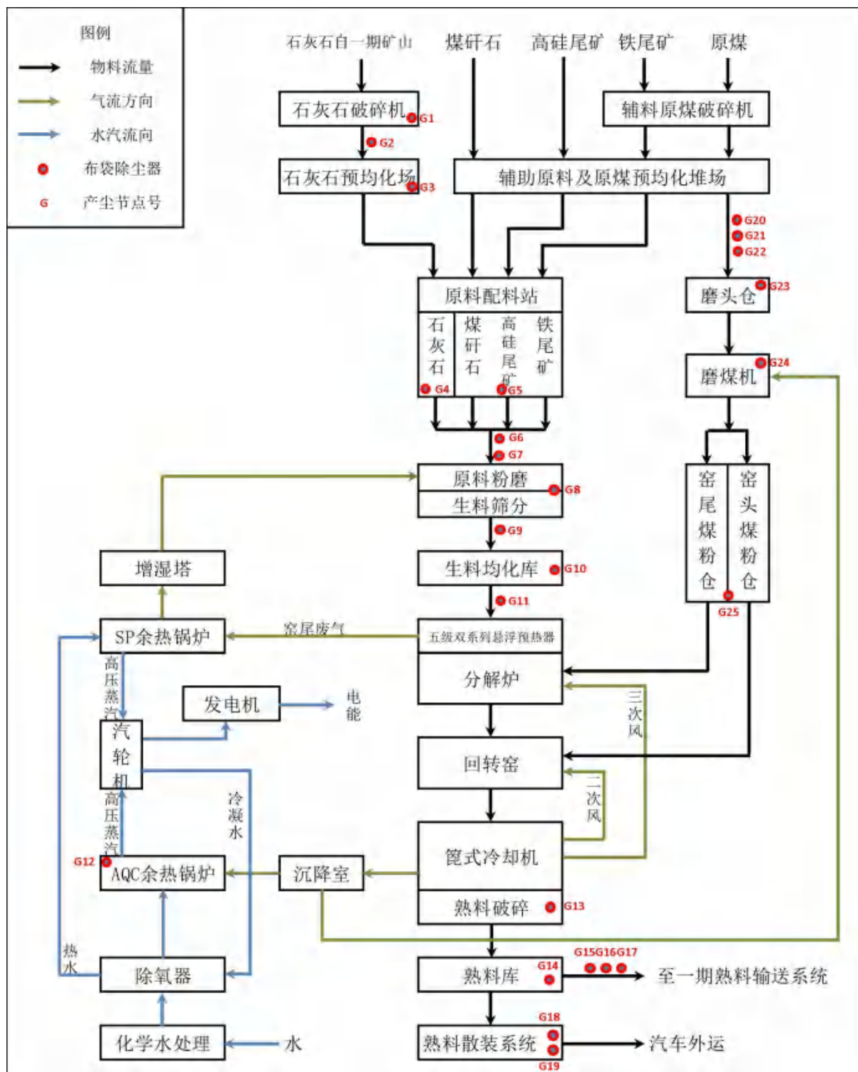
图 3—3 工艺流程及排污节点示意图
